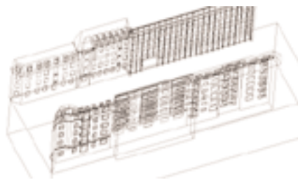
Figure 5 : Modèle filaire issu de la restitution des façades de la rue de l'Argonne (Strasbourg).
