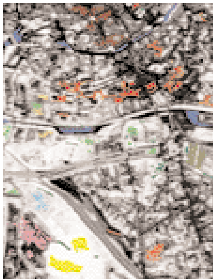
Figure 10 : Echantillons sélectionnés sur le niveau de segmentation 2 (extrait du transect Nord-Sud).
