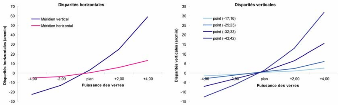
Figure 6 : variation de la disparité horizontale (à gauche) et de la disparité verticale (à droite) en fonction de la puissance des verres étudiés (-4,00 δ ; -2,00 δ ; plan ; +2,00 δ ; +4,00 δ) pour plusieurs points du champ visuel : pour les disparités horizontales, il s'agit de deux points à 43° d'excentricité sur le méridien horizontal (en rose) et sur le méridien vertical (en bleu) ; pour les disparités verticales, ce sont 4 points (dont les coordonnées sont en légende) d'un même quadrant.
