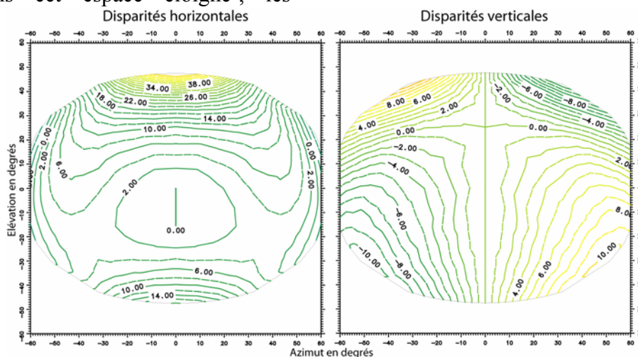
Figure 9 : Cartes d'iso-disparités horizontales (à gauche) et verticales (à droite) pour un couple de verres de +2,00 δ placé devant les yeux selon un angle pantoscopique de 15°.
