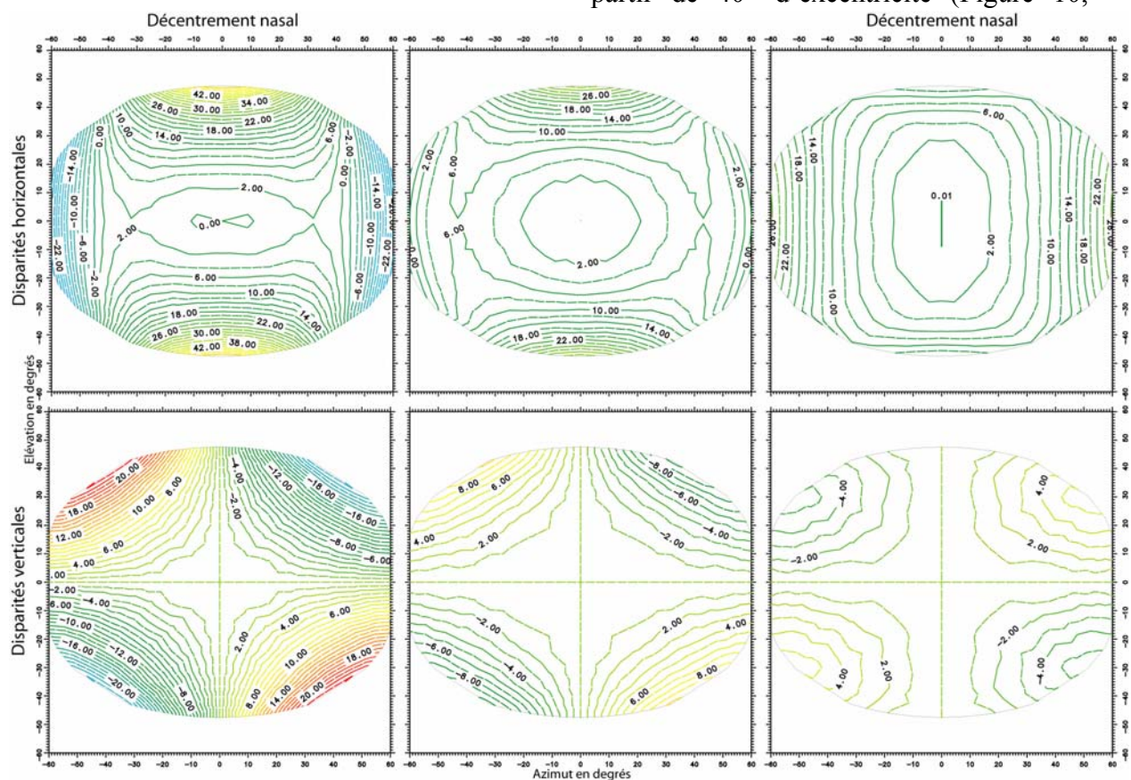
Figure 10 : Cartes d'iso-disparités horizontales (en haut) et verticales (en bas) pour un couple de verres de +2,00 δ, décentrés de 3 mm en nasal pour les deux yeux (à gauche) ou de 3 mm en temporal pour les deux yeux (à droite), le couple de verres correctement centrés se trouvant au centre.
