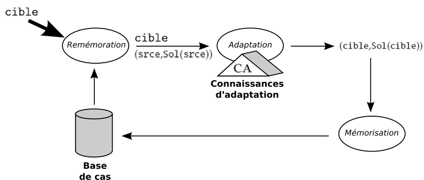
FIG. 1.1 – Schéma général d'un système de RÀPC.
