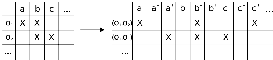
FIG. 2.2 – Construction du contexte d'extraction – Passage du formatage 1 au formatage 2.
