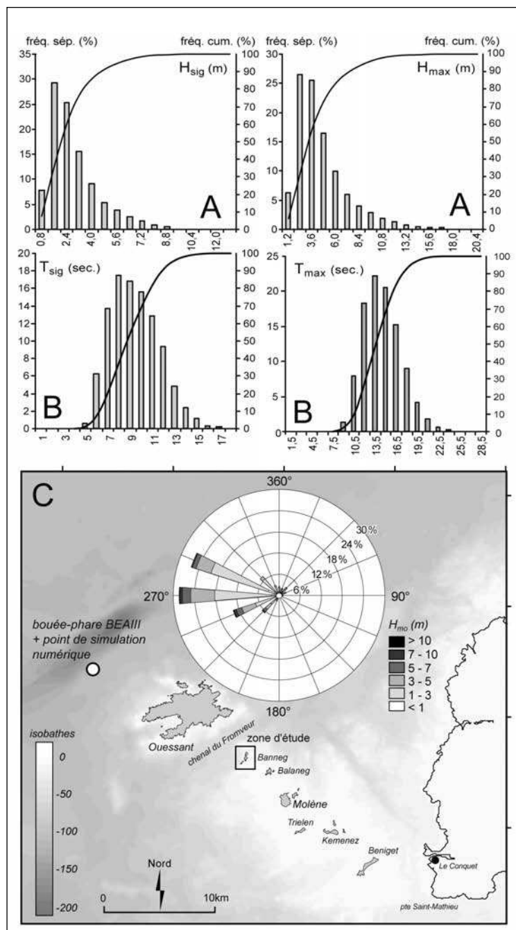
Fig. 3 – Caractéristiques hydrodynamiques de la mer d'Iroise. Histogrammes de houles. A : hauteurs significatives Hsig et hauteur maximale Hmax ; B : périodes significatives Tsig et période maximale Tmax à partir des mesures effectuées au large de Ouessant par la bouée-phare BEAIII du 30/08/1985 au 17/08/2001 (source : site Candhis du CETMEF – http://www.cetmef.equipement.gouv.fr/donnees/candhis/home.php ) ; C : spectre directionnel des houles au large de Ouessant (source : simulations numériques effectuées par le LNHE-EDF avec le soutien du CETMEF).
