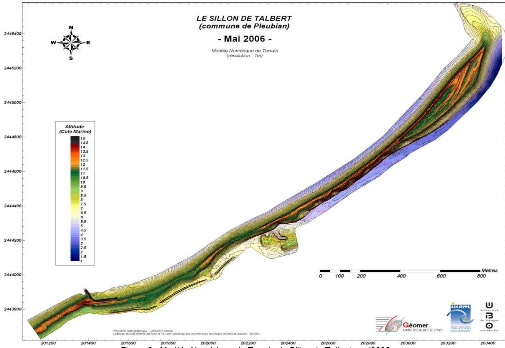
Figure 8 : Modèle Numérique de Terrain du Sillon de Talbert, mai2006.
