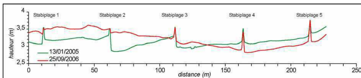
Figure 11 : Evolution du profil longitudinal de la plage recoupant les cinq Stabiplate® dans leur partie médiane entre le mois de janvier 2005 et le mois de septembre 2006
