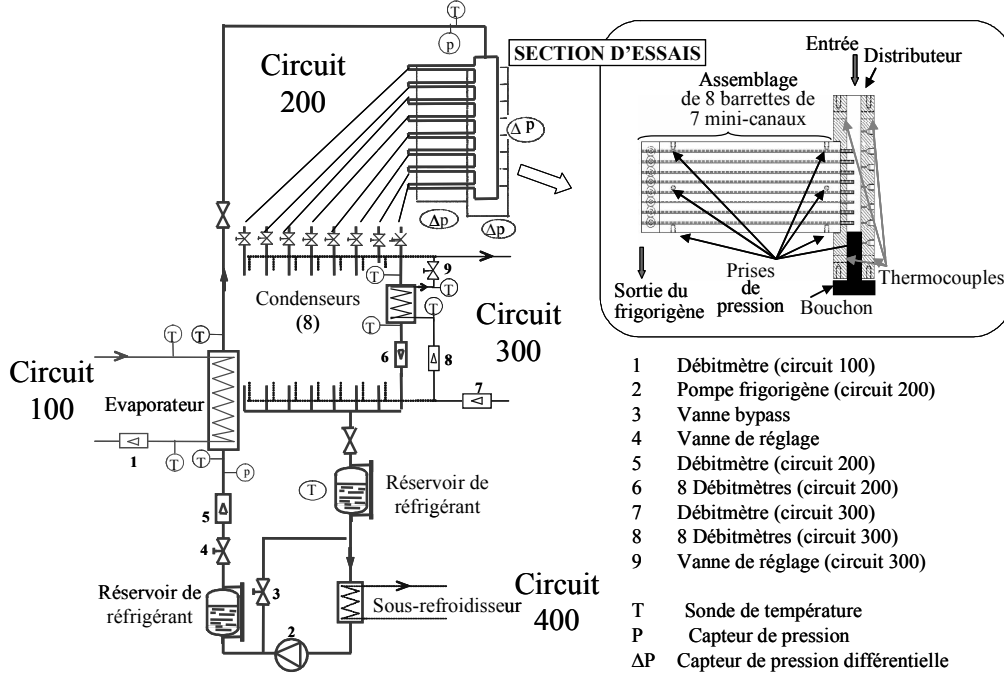
Figure 2 : Dispositif expérimental
