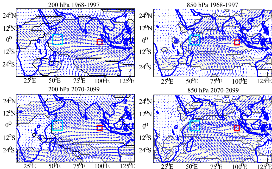
Figure 10. Corrélations [tsmE-tsmW] - vents simulés à 200 et 850 hPa
