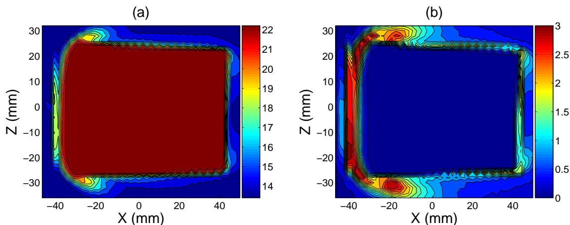
FIG. 1 – Champs de température interpolés sur 50x35 points de mesure à 1 mm de l'entrée du jet. L'écoulement principal arrive du côté gauche de la figure. a) \langle T \rangle b) \theta_{rms} .
