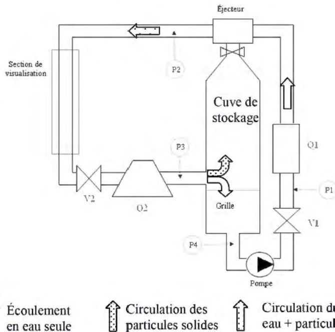
Figure 3 : Schéma du dispositif expérimental
