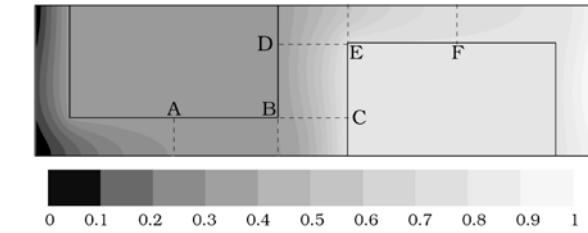
Figure 4 : Chauffage à source volumique uniforme dans les barres. Champ de température adimensionnelle. Domaine de contrôle a de la Fig.1 (réseau en quinconce). Pr = 7 , Re_d = 0.5 , \varepsilon = 0.44 .
