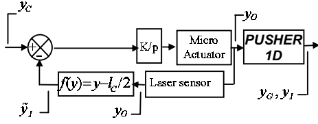
Fig. 14. Right estimator controller.
