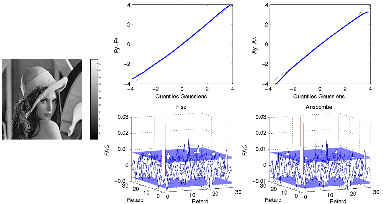
Fig. 1. Comparaison des transformations de Fisz et d'Anscombe sur du bruit Poissonien simulé à partir de deux images des intensités, l'une du fantôme de Hoffman et l'autre de Lena. Pour chaque image, les graphes des quantiles sont sur la 1 ère ligne et les FACS sur la 2 ème ligne. Les plans horizontaux sur les FACs correspondent aux limites de Barlett à 5%.
