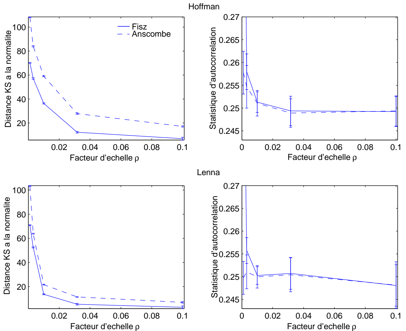
Fig. 2. Comparaison des transformations de Fisz et d'Anscombe sur du bruit Poissonien simulé à partir de deux images des intensités, l'une du fantôme de Hoffman et l'autre de Lena. Pour chaque image, nous avons tracé les graphes de la distance à la normalité (par un test de Kolmogorov-Smirnov) et de la statistique d'auto-corrélation (par un test de Box-Pierce) en fonction du rapport d'échelle simulant différents taux de comptage.
