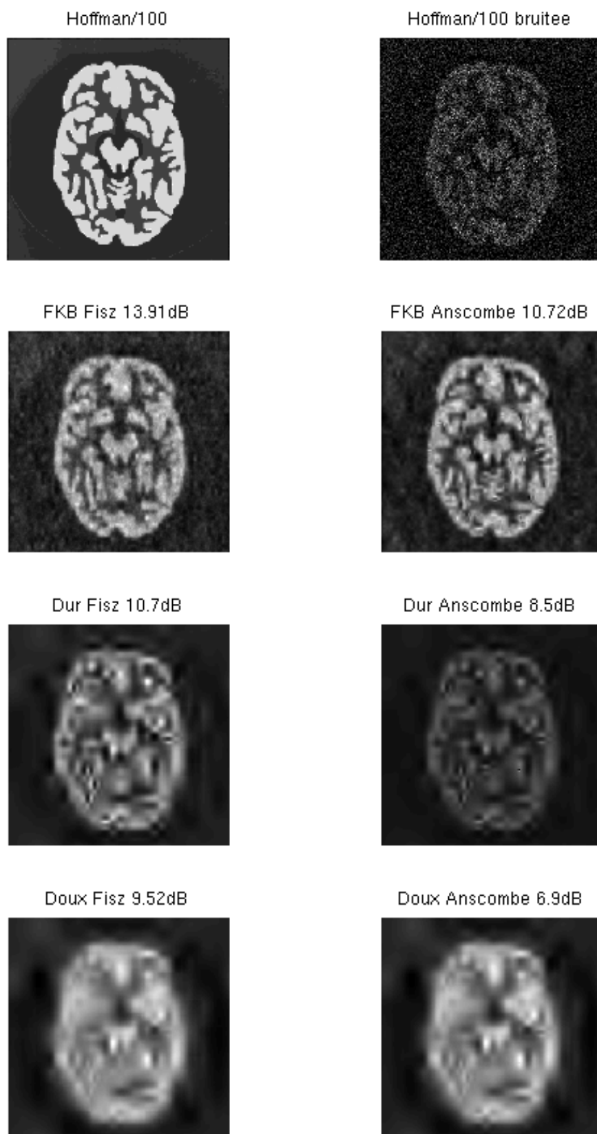
Fig. 3. Exemple d'application des transformées de Fisz (colonne 1) et d'Anscombe (colonne 2) avec les débruiteurs bayésien FKB et universel avec seuillages dur et doux. L'image de Hoffman bruitée est contaminée par un bruit de Poisson après avoir divisé l'image des intensités par 100 (très faible taux de comptage). Les valeurs du RSR sont aussi portés au dessus de chaque image. August 10, 2004
