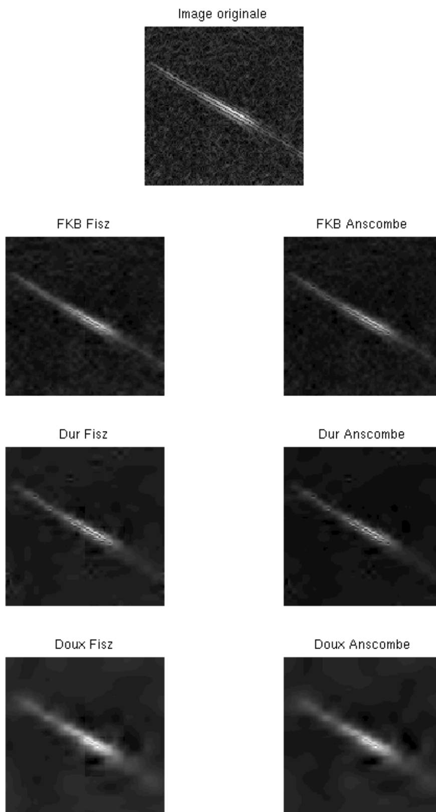
Fig. 5. Comparaison des transformations de Fisz et d'Anscombe avec divers débruiteurs sur une image réelle d'un défaut obtenue par imagerie magnéto-optique. La première image est l'image des comptages originale. Les autres correspondent aux résultats après transformation de Fisz ou d'Anscombe, débruitage (FKB, seillages dur ou doux) puis transformation inverse.
