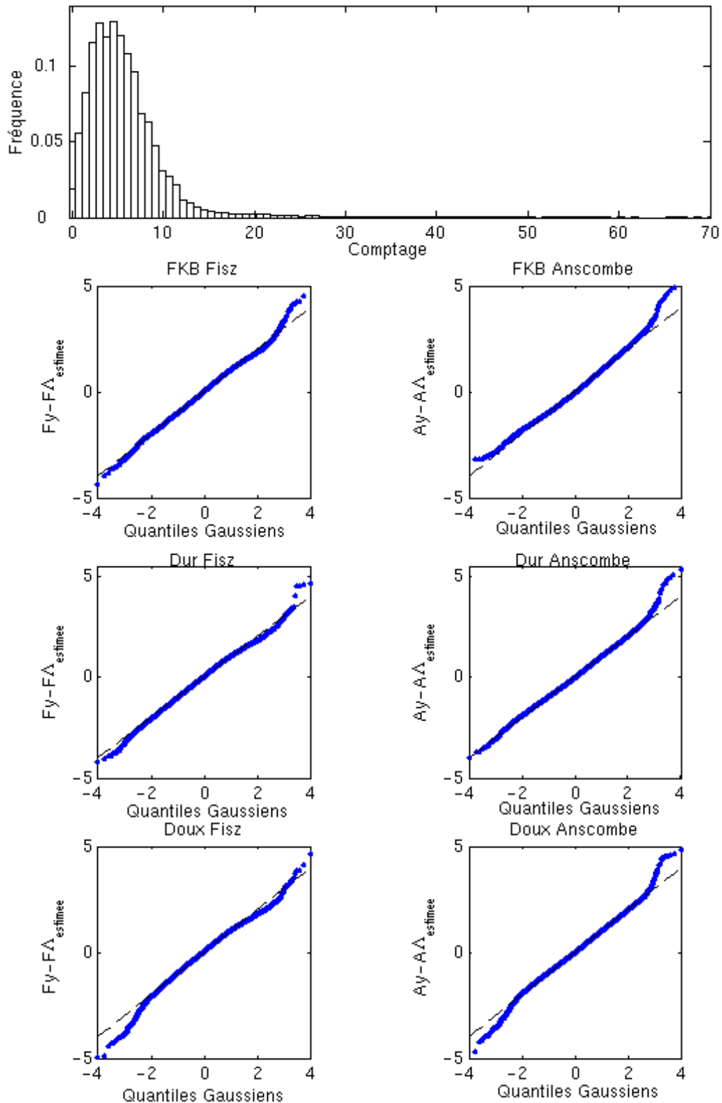
Fig. 6. Tracés des résidus entre la transformée de l'image originale ( \mathcal{F}\mathbf{y} ou \mathcal{A}\mathbf{y} ) et celle de sa version débruitée ( \widehat{\mathcal{F}\Lambda} ou \widehat{\mathcal{A}\Lambda} ), en fonction des quantiles gaussiens. Le premier graphe montre l'histogramme de l'image originale avec un mode important à faible taux de comptage correspondant au fond. Les graphes suivants correspondent aux tracés des quantiles pour les résidus obtenus par chaque débruiteur (FKB, seuillages dur ou doux) dans le domaine de chaque transformation, de Fisz ou d'Anscombe.
