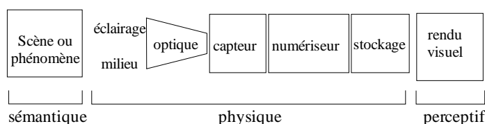
Fig. 4. Le schéma de principe d'une acquisition d'images définit les différents catégories d'informations à renseigner pour formuler un modèle du domaine.
