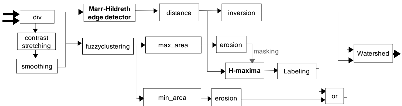
Fig. 11. Un programme est un graphe d'exécution d'opérateurs codés comme des programmes exécutables. Le programme ci-dessus permet de localiser les noyaux de cellules de séreuse. Il prend en entrée une image de séreuse et une image de champ optique vide et retourne une carte de régions localisant les noyaux de séreuse. "Marr-Hildreth edge detector" et "H-maxima" sont des procédures composées de plusieurs opérateurs. La sortie de l'érosion est utilisée comme masque de la procédure H-maxima.
