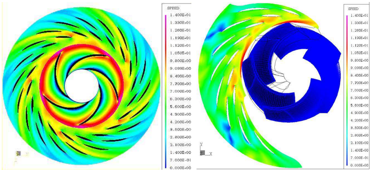
A) Q=1.17Q_n .
