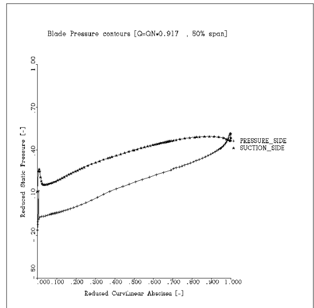
B) Q=0.9Q_n
