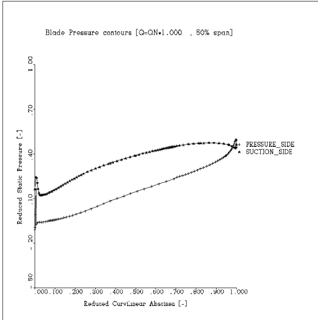
C) Q=Q_n .
