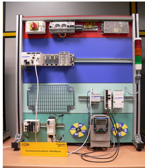
Figure 3. Modbus module
