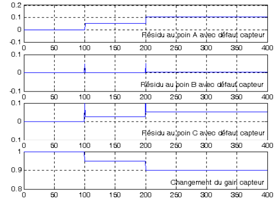
Figure 5 : Résidus aux points A, B et C pour un changement du gain du capteur K_s .
