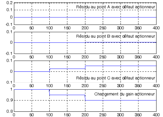
Figure 4 : Résidus aux points A, B et C pour un changement du gain de l'actionneur K_a .
