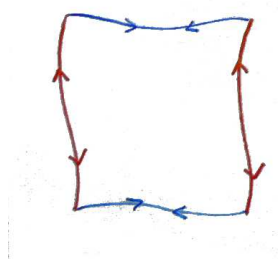
FIGURE 1. Un carré borné par quatre courbes alternativement incluses dans \mathcal{F}^s et \mathcal{F}^u .
