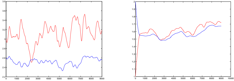
Figure 3. Entrées u_1(t) (en clair) et u_2(t) (en foncé). Figure 4. Sorties y_1(t) (en clair) et y_2(t) (en foncé).
