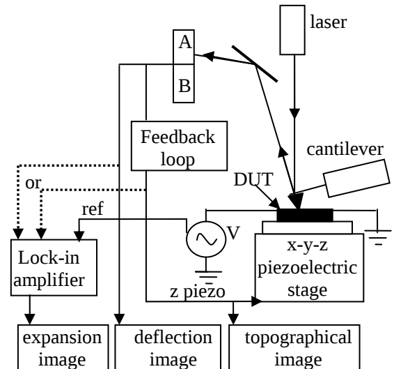
Fig. 1: SJEM set-up
