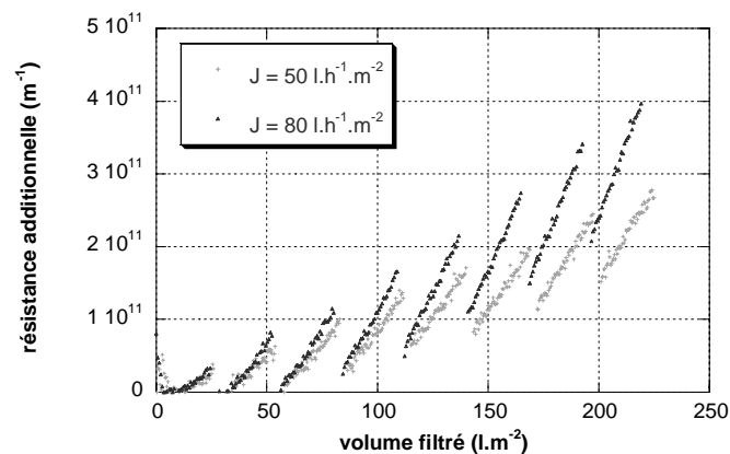
Figure 6 : mise en œuvre de purges dans une filtration « subcritique » - volume filtré entre purges V_f=25 \text{ l.m}^{-2}
