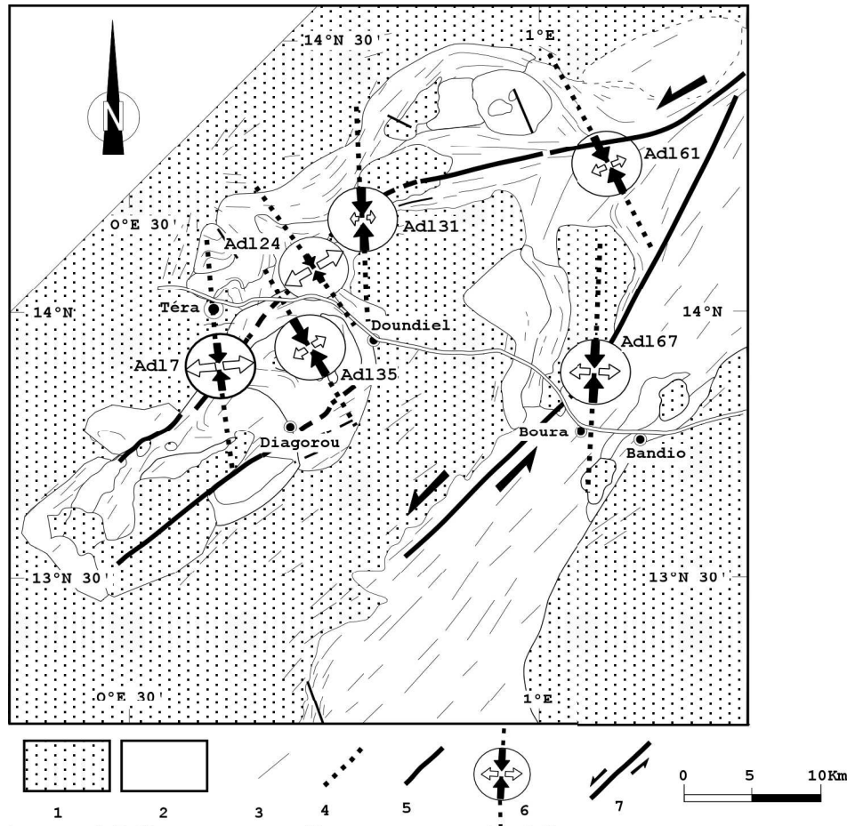
Figure 10. Champ de paléocontraintes relié à l'épisode de déformation relativement cassante D1c à raccourcissement N345 à N10°E; 1: Granitoides variés; 2: Ceinture de roches vertes; 3: Trajectoire de la foliation /schistosité S1; 4: Faille supposée ou contact tectonique; 5: Couloir de déformation majeur; 6: Trajectoires de contraintes \sigma_1 reliés à la phase D1c; 7 : Réactivation sénestre des accidents N45°E.
