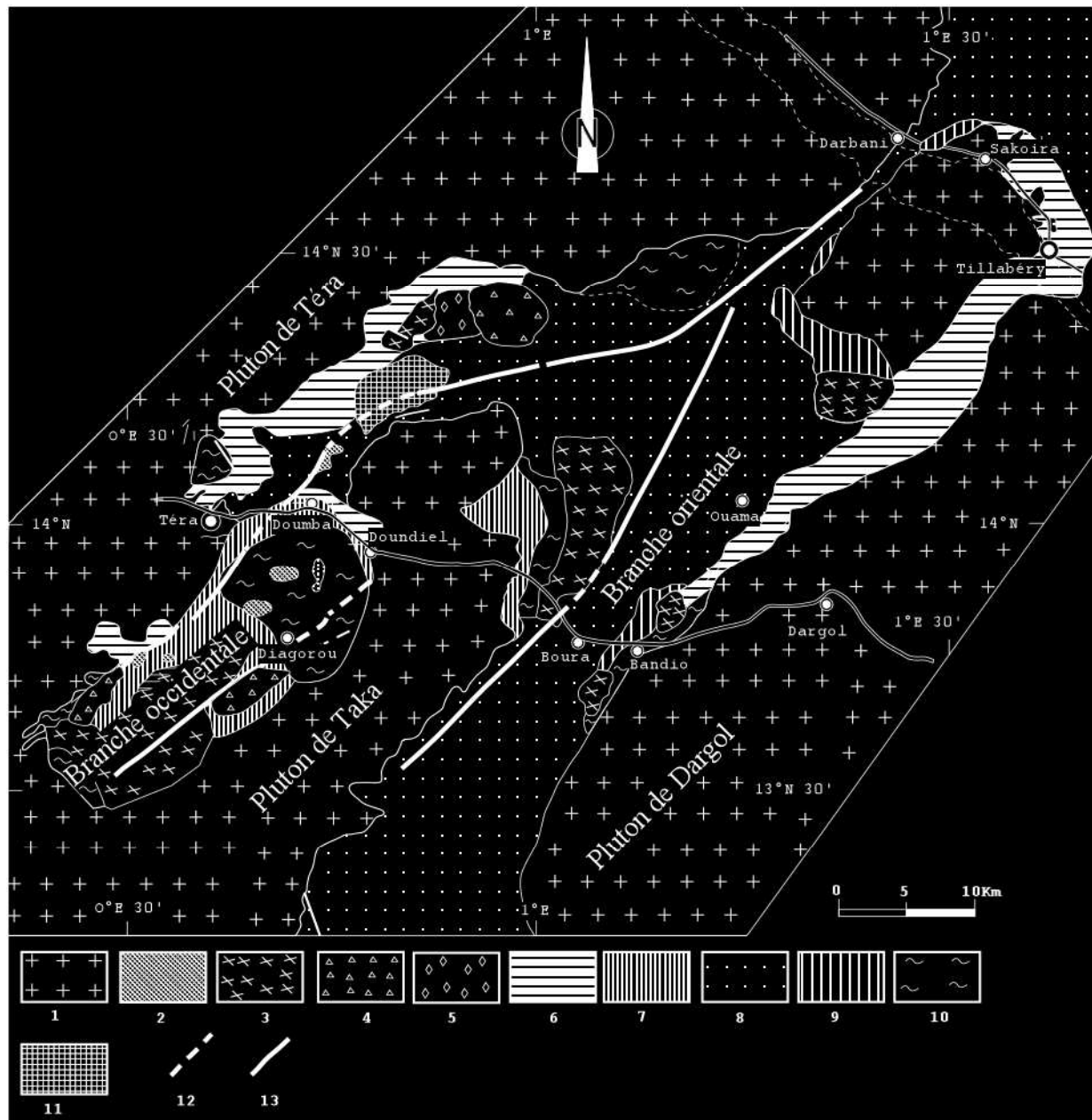
Figure 2. Carte géologique de la ceinture de Diagorou-Darbani (d'après Soumaila, 2000; modifiée)
