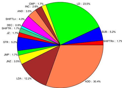
FIG. 2: Taux d'utilisation des différents opérateurs pour le démosaïquage par interpolation bilinéaire.
