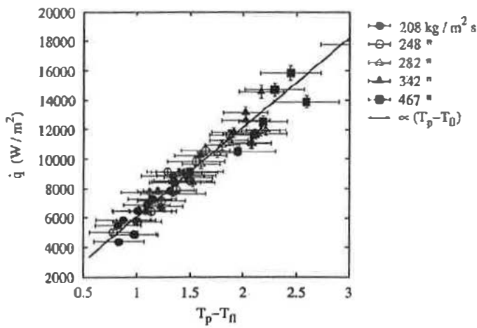
Figure 3 : T_p - T_{fl} en fonction de \dot{q} , x = 0,3 , D_h = 0,77 mm
