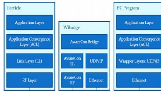
Fig. 3. La connexion entre la Particule et le PC
