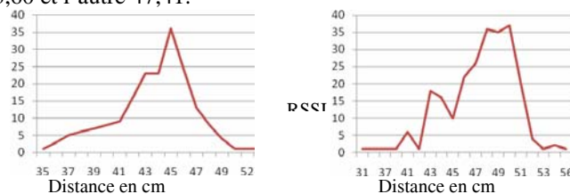
Fig.10. Indications RSSI pour deux particules positionnées à 100 cm une de l'autre
