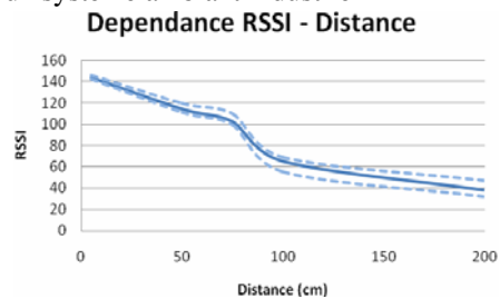
Fig. 8. La dépendance entre le RSSI et la distance
