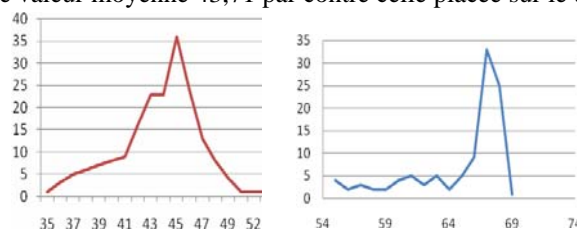
Fig. 9. Indications RSSI pour différentes positions des pParticules (gauche – particule sur terre et droite – particule sur le bureau)
