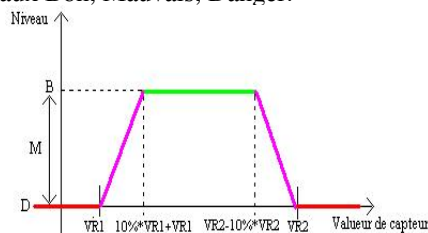
Fig. 4. Les niveaux de sécurité ambiante
