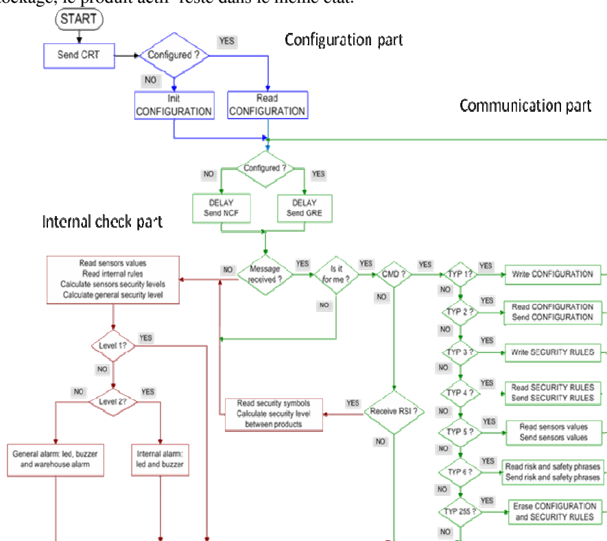
Fig. 6. Modèle Algorithmique Interne du Produit Actif
