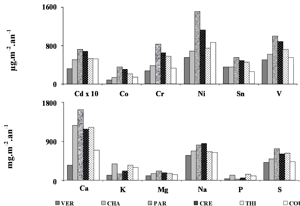
Figure 4. Flux annuels ( \mu\text{g.m}^{-2}.\text{an}^{-1} ) des retombées atmosphériques d'éléments minéraux sur la région parisienne.
