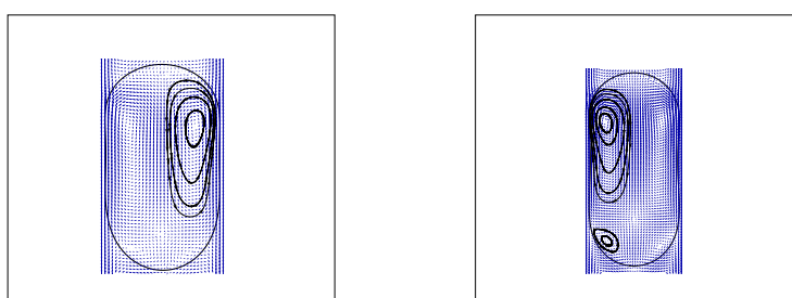
FIG. 5 – A gauche : données de référence sauf que u_{in} = 0.05 m/s. A droite : données de référence avec une goutte encore plus grosse et une vitesse faible (voir texte).
