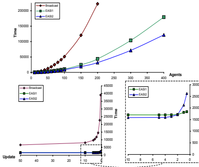
FIG. 3 – Broadcast - Algorithmes EASI. Temps d'exécution en fonction du nombre d'agent (haut) et du taux de mise à jour (bas).
