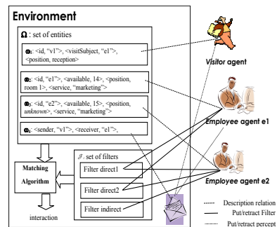
FIG. 1 – Exemple de modélisation des interactions avec EASI
