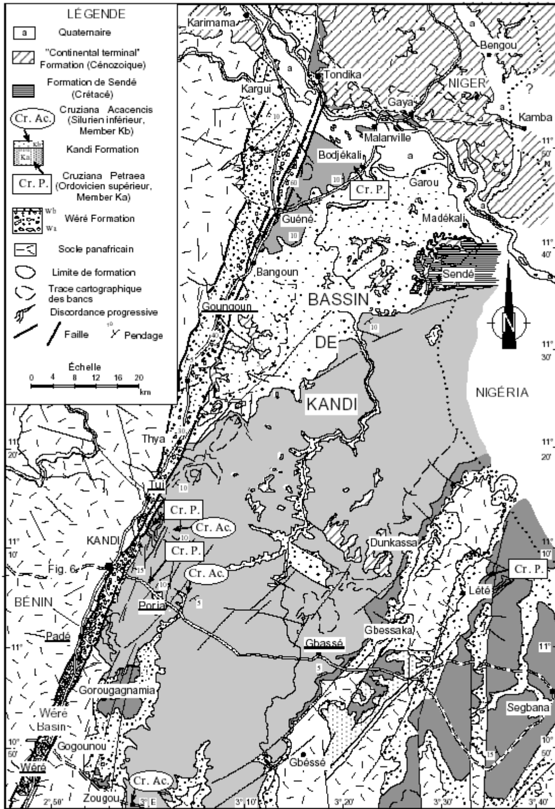
Figure 5. Carte géologique générale du bassin de Kandi (Konaté, 1996).
