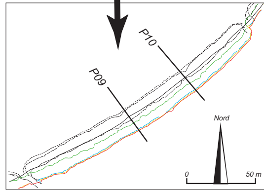
[7] Évolution du front de dune de la partie orientale de la plage du Vougot entre 1952 et 2006, avec un zoom sur la période 2004-2006 obtenu par la mesure de terrain au DGPS. Les vitesses de recul enregistrées durant ces 3 dernières années avoisinent 1 m/an.
