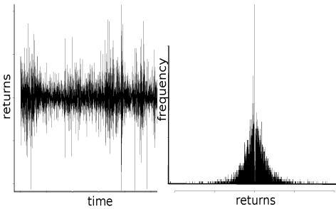
FIG. 1 – Rendements journaliers du titre BMW et leur distribution
