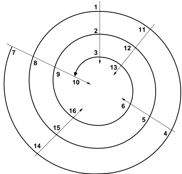
FIGURE 8. La 5-pérecquine de 16
