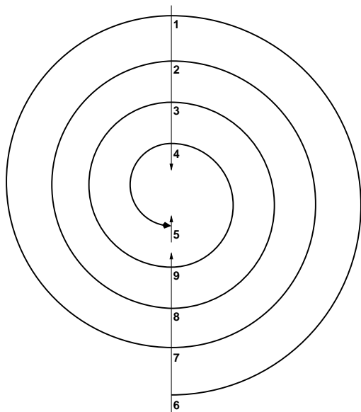
FIGURE 9. La 2, 10-pérecquine de 9
