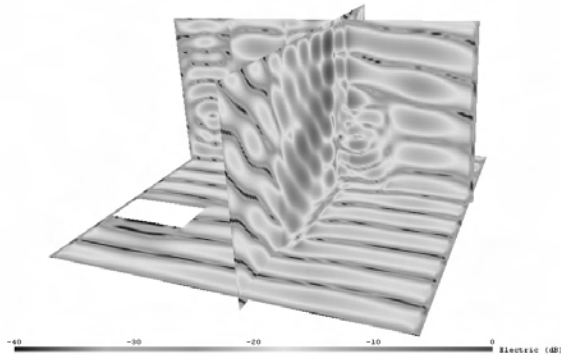
Figure 12 : Application "télévision 500 MHz"
