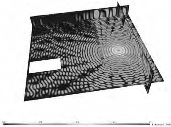
Figure 13 : Application "téléphonie 1800 MHz"
