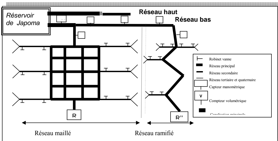
Figure 1 : Structure du réseau de distribution d'eau à Douala
