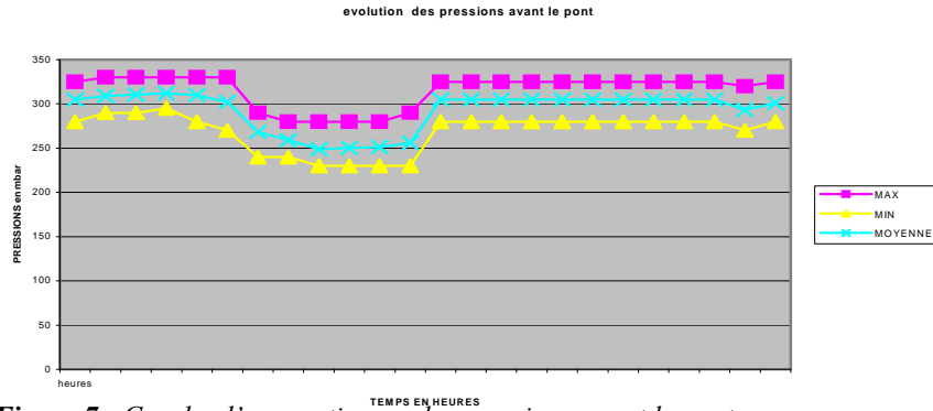
Figure 7 : Courbe d'apprentissage des pressions avant le pont
