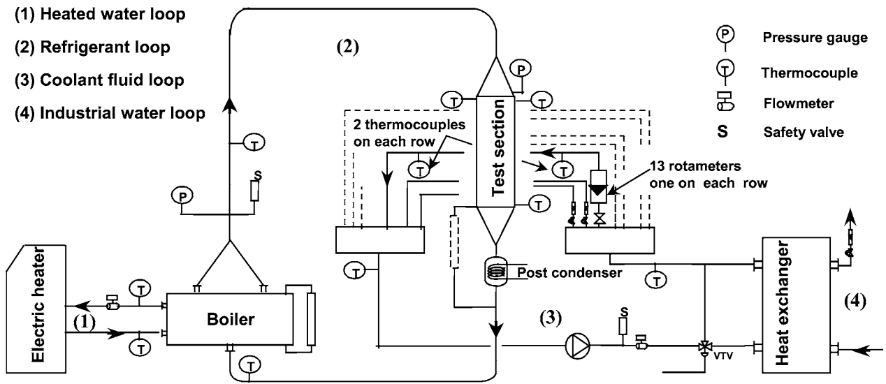
Fig. 1. Test rig.
