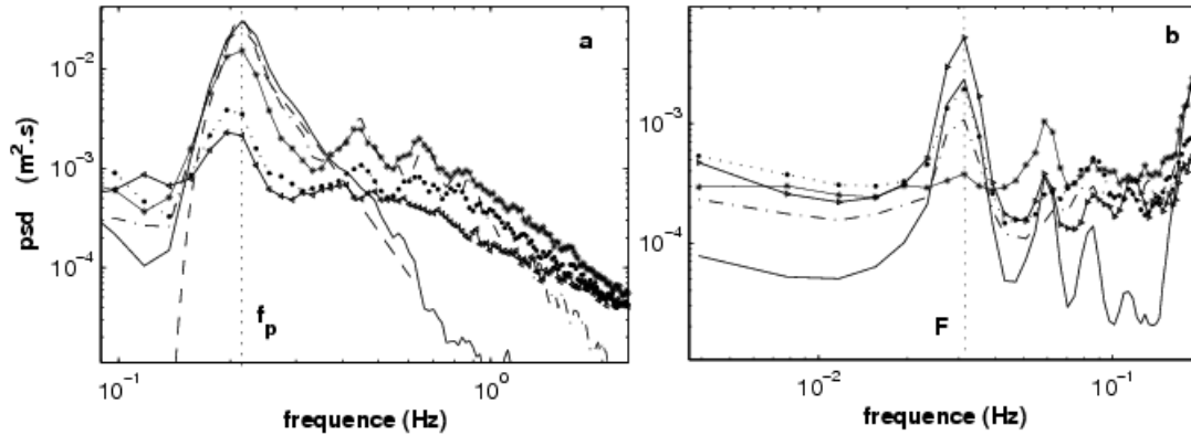
Figure 2- Evolution des spectres d'énergie. a- Spectre de consigne (---), les spectres mesurés à x=1,77 \text{ m} (---), à x=9,47 \text{ m} (-), à x=14,47 \text{ m} (-*), à x=21,97 \text{ m} (-•) et à x=24,47 \text{ m} (<) du batteur. b- Les spectres mesurés dans la zone basse fréquence. Consigne: H_{rms}=11,31 \text{ cm} , f_p=0,2116 \text{ Hz} , h_0=60 \text{ cm} (expérience-40).
