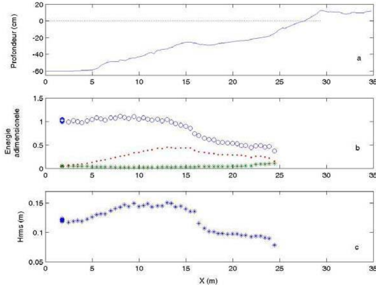
Figure 3- a. Profil de fond. b. Energie totale (o), Energie basse fréquence (*) et Energie des différents harmoniques (.) mesurées en chaque point et rapportées à celle de la première sonde située à 1,77m du batteur. c. Evolution des H_{rms} . Consigne: H_{rms}=11,31cm , f_p=0,2116Hz , h_0=60cm , largeur de spectre: 0,6 f_p < f < 2,4 f_p (expérience-40).
