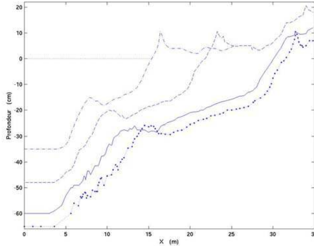
Figure 4- H_{rms}=8cm, f_p=0,33Hz, h_0=35cm , expérience-29: (-), H_{rms}=9,88cm, f_p=0,27Hz, h_0=48cm , expérience-36: (- -), H_{rms}=9,88cm, f_p=0,2327Hz, h_0=60cm , expérience-39: (- - -), H_{rms}=12,09cm, f_p=0,2206Hz, h_0=65cm , expérience-41: (- •), largeur de spectre de consigne: 0,6 f_p < f < 2,4 f_p .
