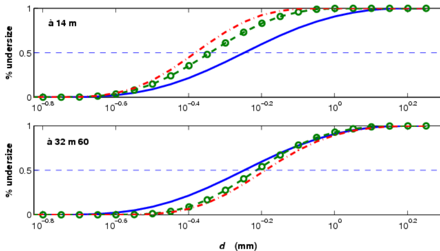
Figure 8- Distribution granulométrique en 2 sections au début (O) et à la fin de l'expérience-3 (.-)(après 13h30), (consigne: H_{ms}=12,3\text{cm} , f_p=0,4\text{Hz} , h_0=65\text{cm} , largeur de spectre: 0,8f_p < f < 1,8f_p ), comparée à la distribution moyenne (---).
