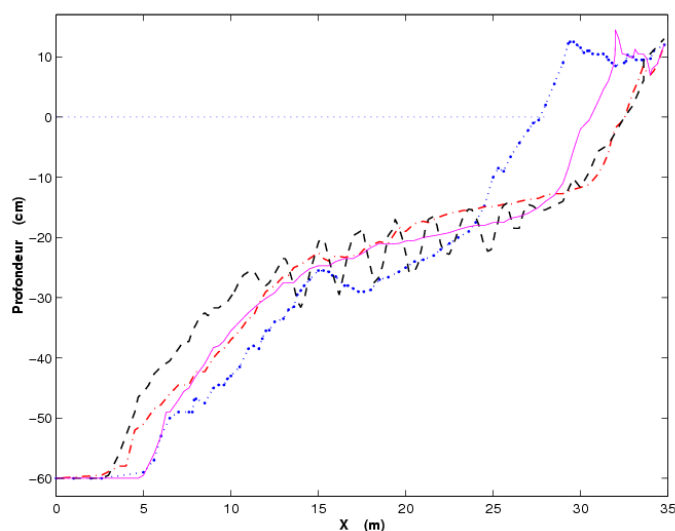
Figure 6- Expérience-44 ( \Omega=2,76 ): (---), expérience-38 ( \Omega=2,12 ): (- -), expérience-40 ( \Omega=1,92 ): (-●-), expérience-43 ( \Omega=1,71 ): (-.).
