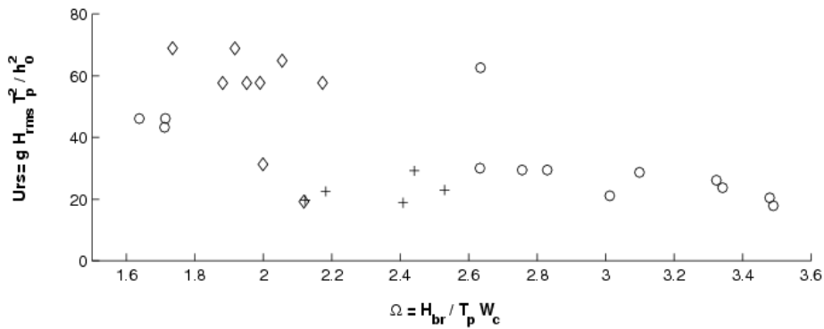
Figure 5- Plage terrasse: (O), Plage multi-barres (en évolution rapide): (+), Plage-barrée: (◇).
