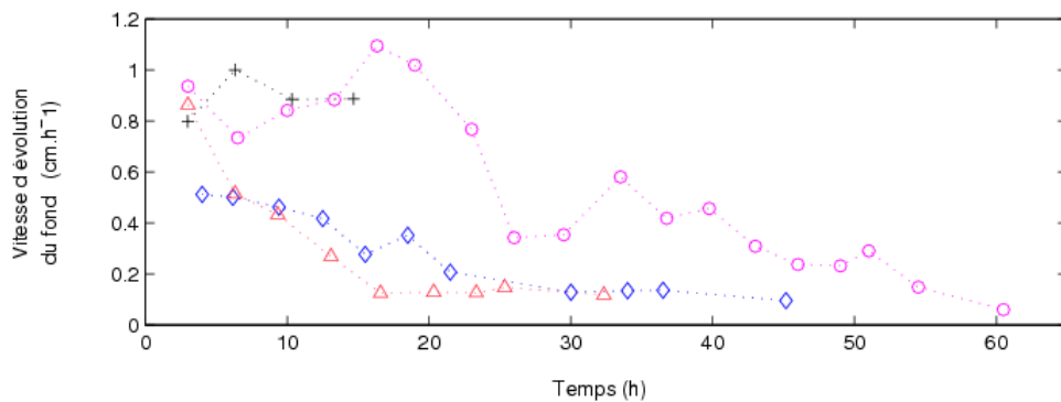
Figure 7- Vitesse de l'évolution de fond. Expérience-44:( O ), expérience-38:(+), expérience-40:(◇), expérience-43:(△).
