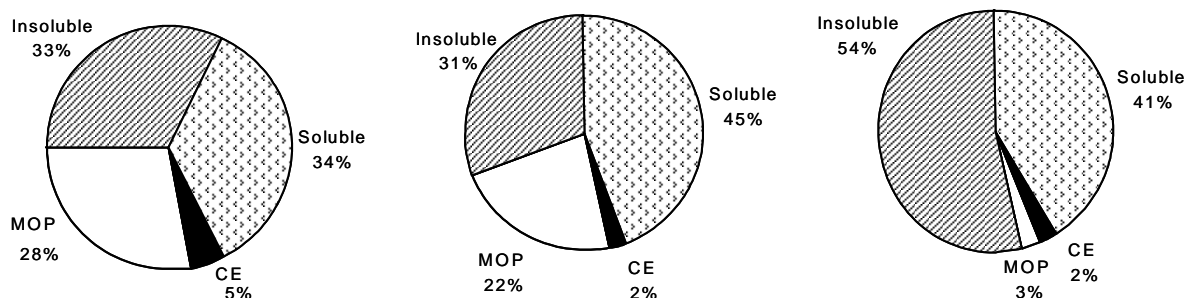
Figure 6 : Pourcentage des différentes fractions constituant l'aérosol (à gauche), le verre à vitres (au centre) et le verre autonettoyant (à droite) ; (CE : carbone élémentaire, MOP : matière organique particulaire).
