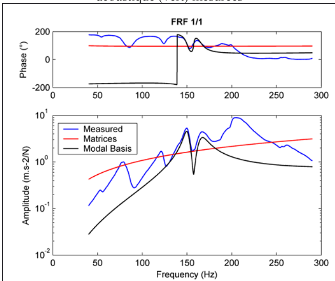
Figure 4 : cas de la harpe, FRF vibratoire mesurée (bleu), synthétisée à partir des matrices M, B, K (rouge), synthétisée à partir de la base modale complexe (noir)
