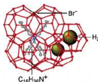
Figure 10 : Représentation structurale du clathrate H_2-TBABr-H_2O
