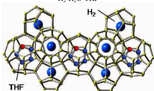
Figure 9 : Représentation structurale du clathrate H_2-H_2O-THF
