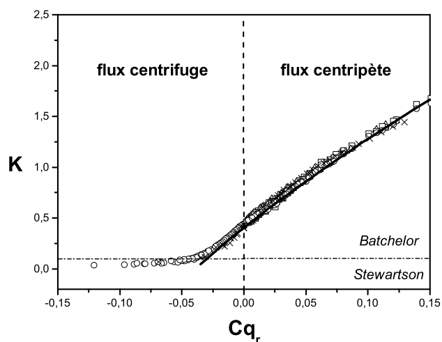
FIG. 6 – Loi K - Cq_r pour différents rapports d'aspect : (\times) G = 0.012 , (\triangle) G = 0.024 , (\circ) G = 0.036 , (\square) G = 0.048 , (-) loi (1).
