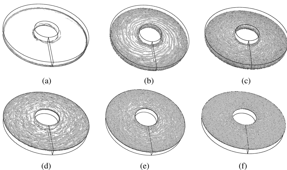
FIG. 7 – Vue de dessus des iso-surfaces du critère Q dans la couche limite du rotor (a,b,c) et dans celle du stator (d,e,f) pour Re = 10^5 (a,d), Re = 4 \times 10^5 (b,e) et Re = 10^6 (c,f).
