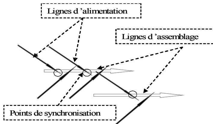
Figure 2: Organisation de la ligne selon la DFT
