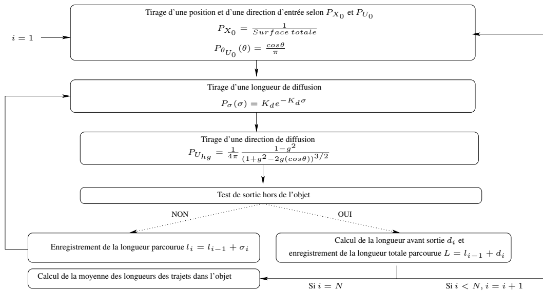
FIG. 1 – Algorithme analogue de diffusions multiples dans une géométrie donnée, pour des fonctions de phase d'Henye-Greenstein avec détail des fonctions de densité de probabilités utilisées.
