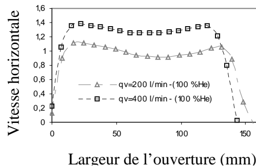
Figure 4 : Profil de vitesse horizontale au niveau de l'ouverture ( q_v : Débit d'injection)
