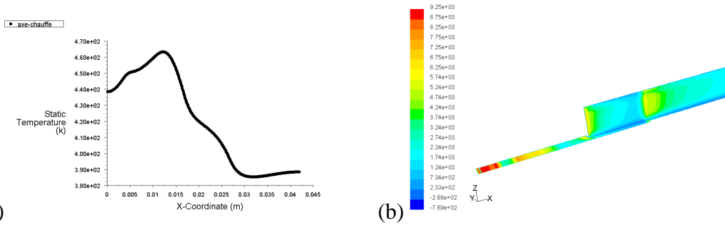
Figure 4 : Profil de température des cellules photovoltaïques (a) et coefficients d'échange thermiques le long du canal (b) pour une vitesse d'entrée de 0,5 m/s
