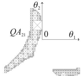
Fig. 12: Free Q-aspect QA_{21}
