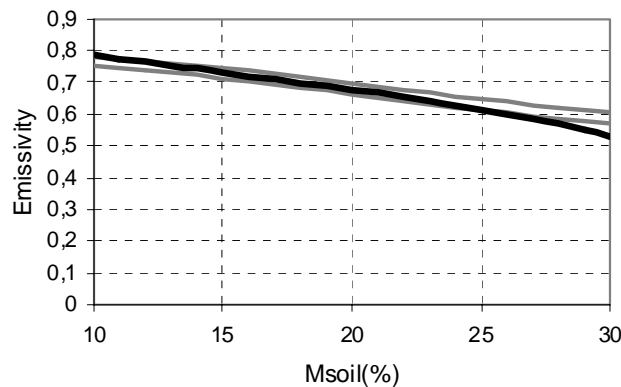
Figure 2 : Emissivité du sol par la méthode \tau-\omega en noir et emissivité du sol via HFSS en gris
