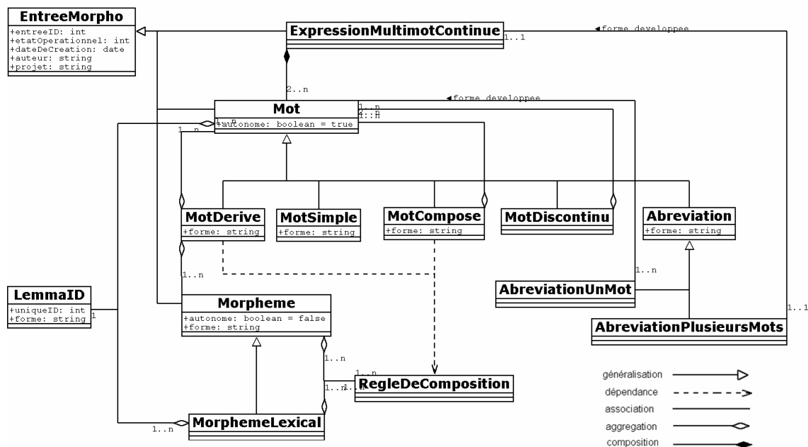
Figure 1 : L'objet Mot et les objets liés
