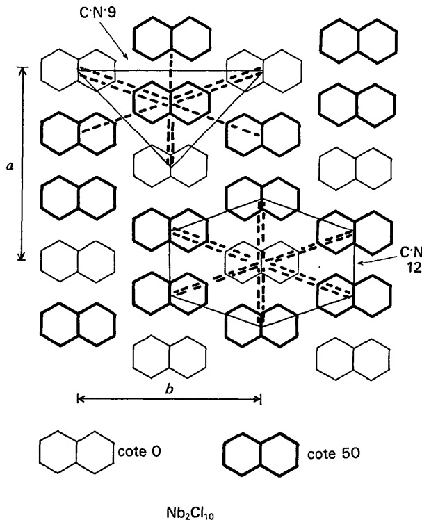
Fig. 3. Schématisation de la structure de NbCl_5 .
