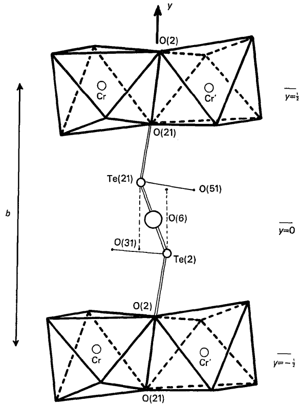
Fig. 2. Connexion de deux groupes (Cr_2O_{10})^{14-} par le groupe (Te_2O)^{6+} selon l'axe Oy .
