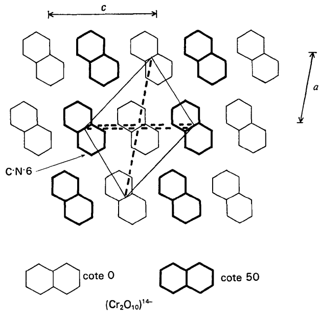
Fig. 4. Schématisation de l'arrangement tridimensionnel des anions (Cr 2 O 10 ) 14- dans la structure de Cr 2 Te 4 O 11 .
