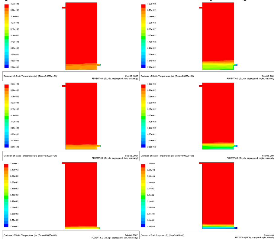
Figure 2 : Comparaison des isothermes après 1 minute dans le cas d'un écoulement laminaire (à gauche) ; débit = 0,045 Kg/s avec ceux trouvées dans le cas d'un écoulement turbulent (à droite) débit = 0,16 Kg/s (droite) pour différentes positions h ( h = 0,05 , h = 0,03 , h = 0 ) de haut en bas.
